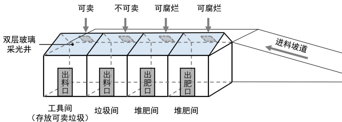
图 6 阳光堆肥房结构图
